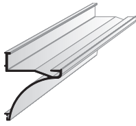
02.0023 Perfil Big Classic
